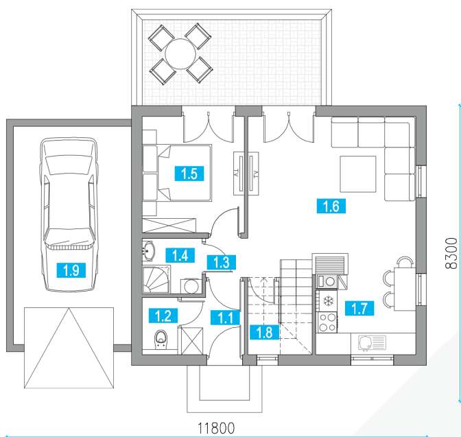
Půdorys přízemní
